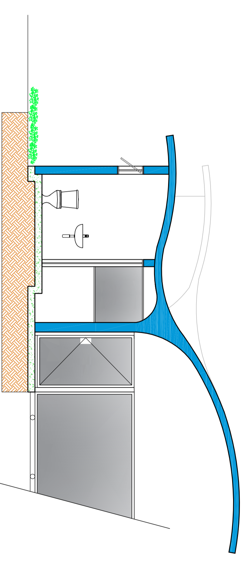
GUARITA CORTE B-B ESC. 1/30 ESCALA GRÁFICA
