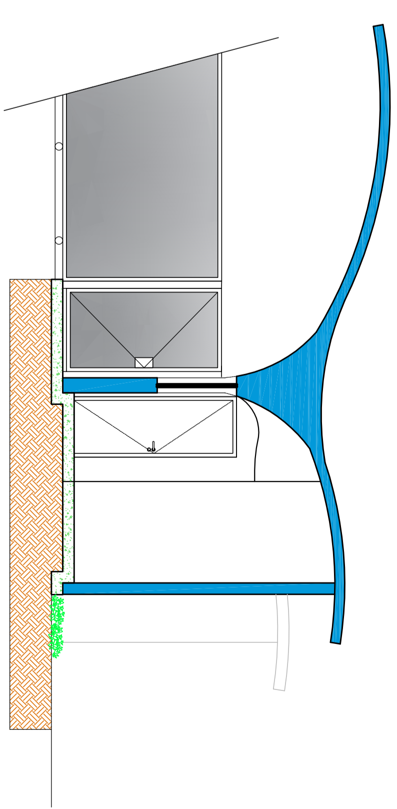
GUARITA CORTE C-C ESC. 1/30 ESCALA GRÁFICA
