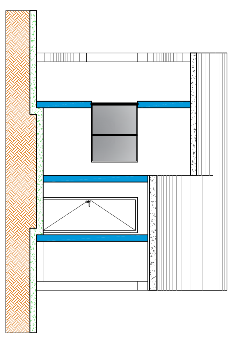
GUARITA CORTE A-A ESC. 1/30 ESCALA GRÁFICA
