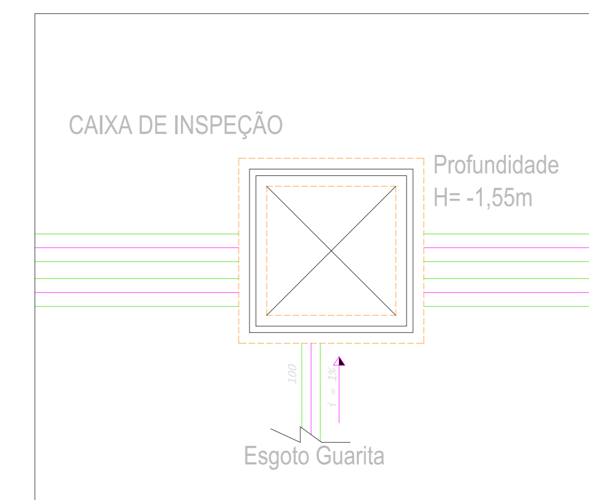
REDE DE ESGOTO DETALHE 24 ESC. 1:20
