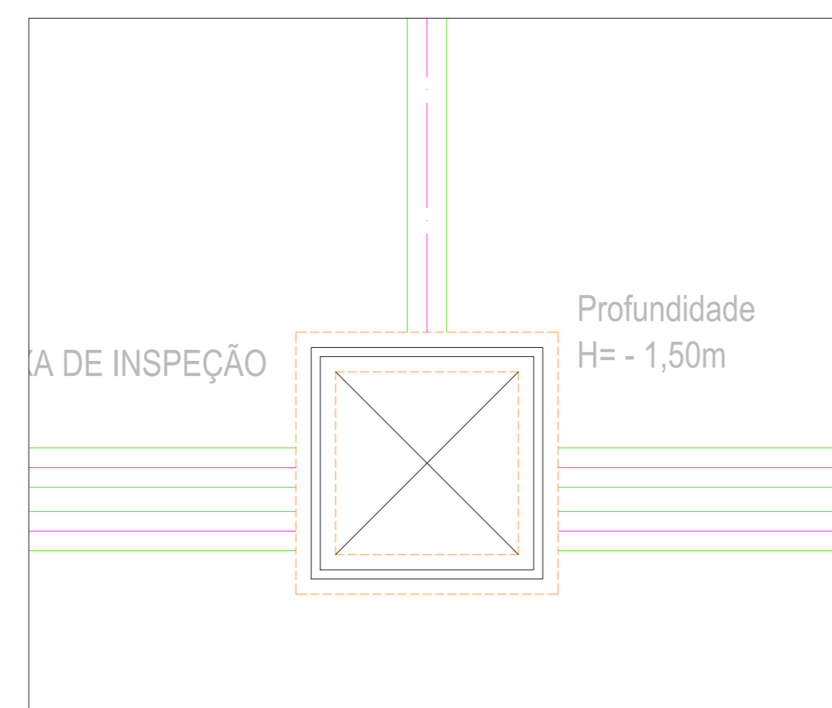
REDE DE ESGOTO DETALHE 19 ESC. 1:20
