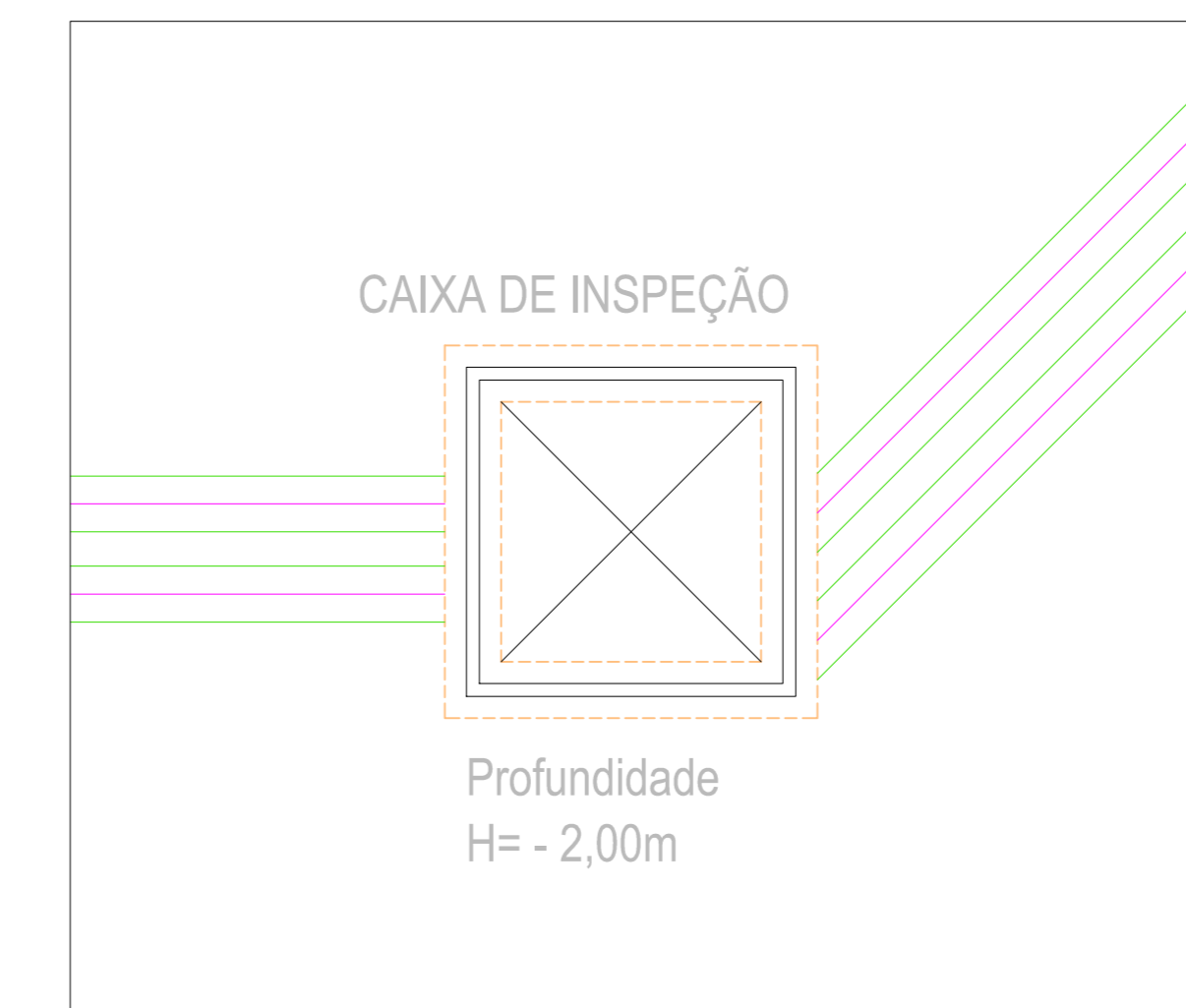
REDE DE ESGOTO DETALHE 22 ESC. 1:20
