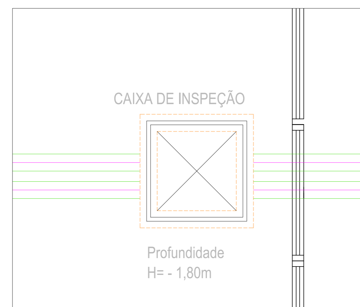
REDE DE ESGOTO DETALHE 21 ESC. 1:20
