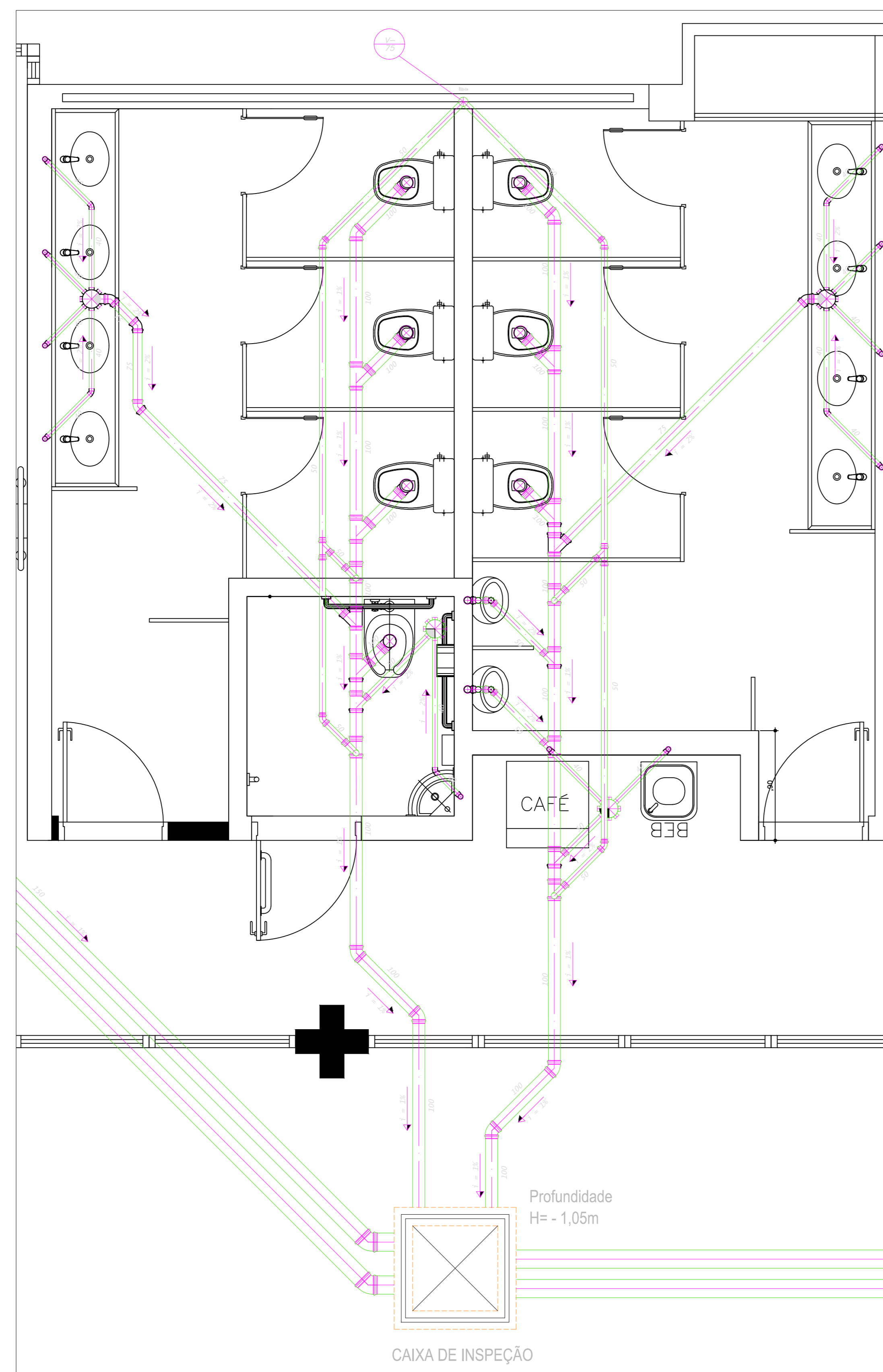
REDE DE ESGOTO DETALHE 13 ESC. 1:25
