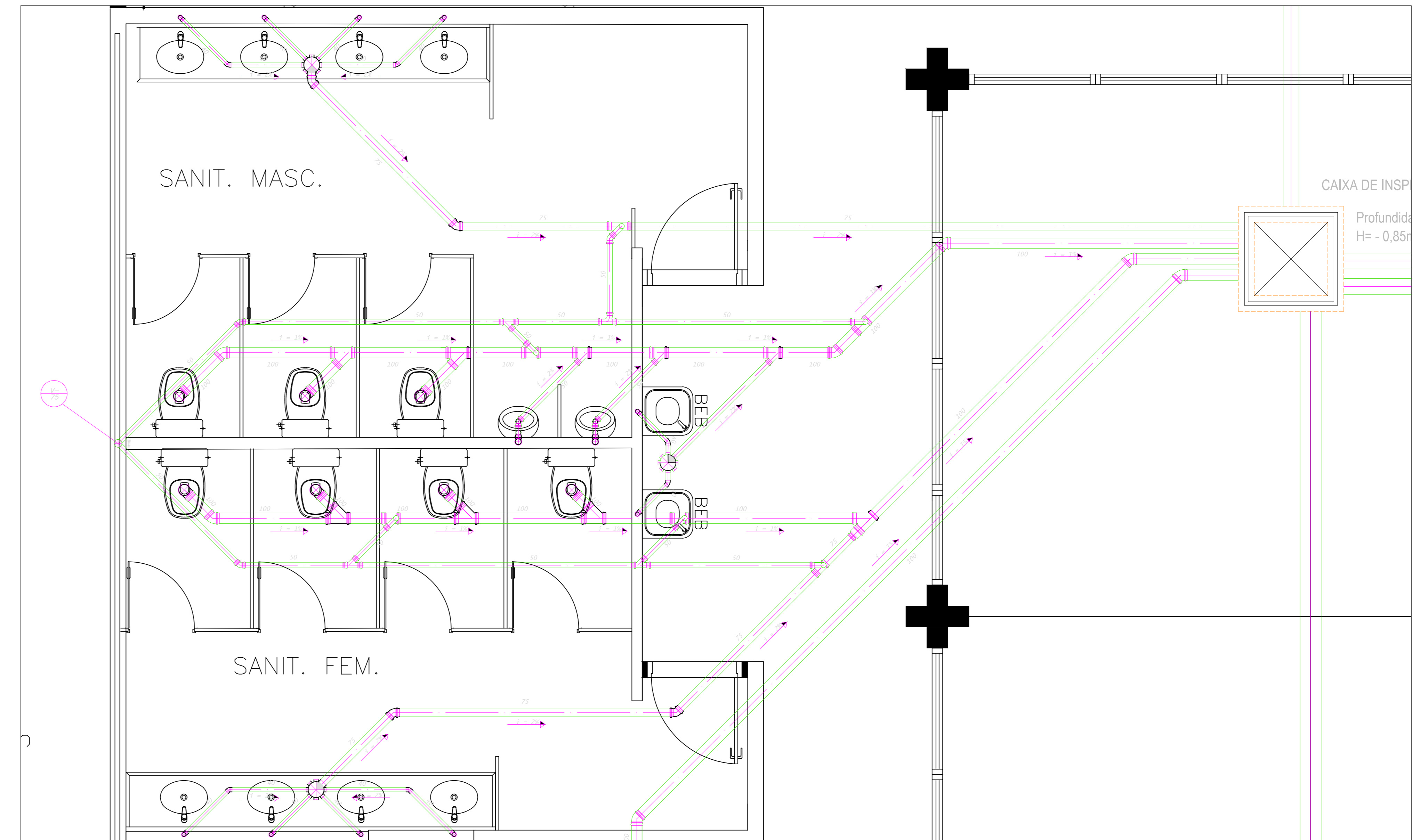
REDE DE ESGOTO DETALHE 12 ESC. 1:25
