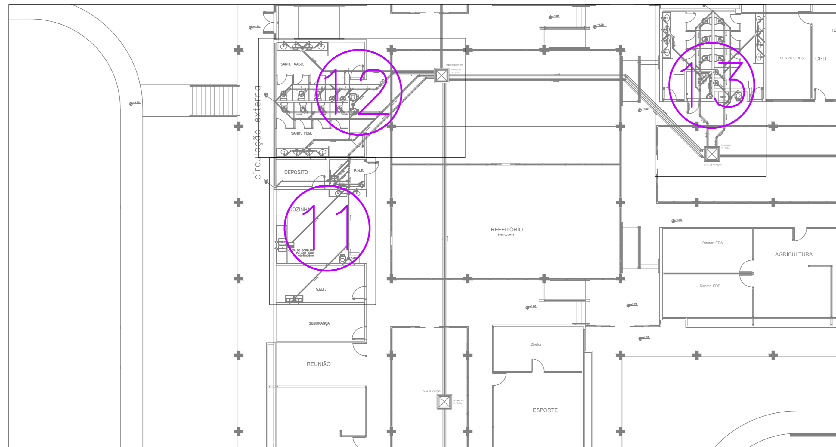
REDE DE ESGOTO GERAL ESC. 1:150
