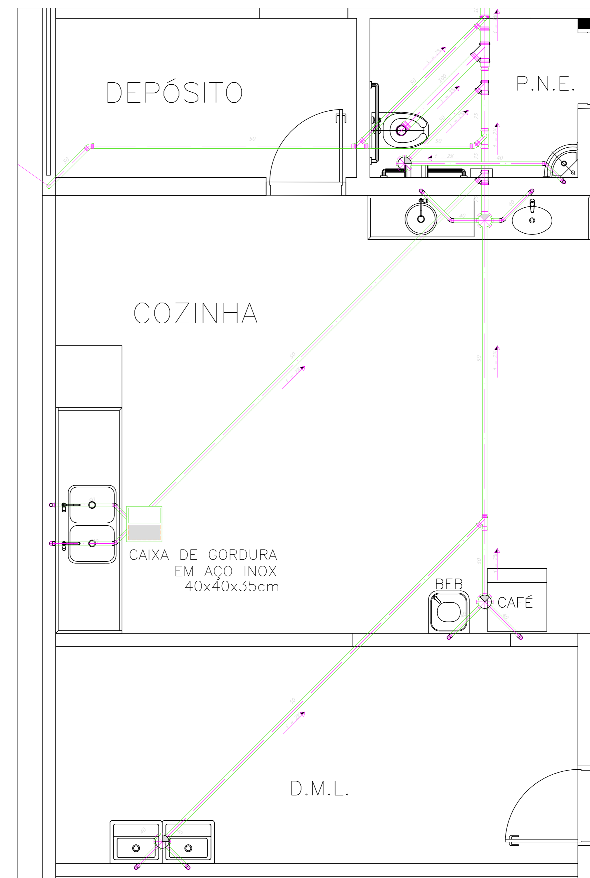
REDE DE ESGOTO DETALHE 11 ESC. 1:25
