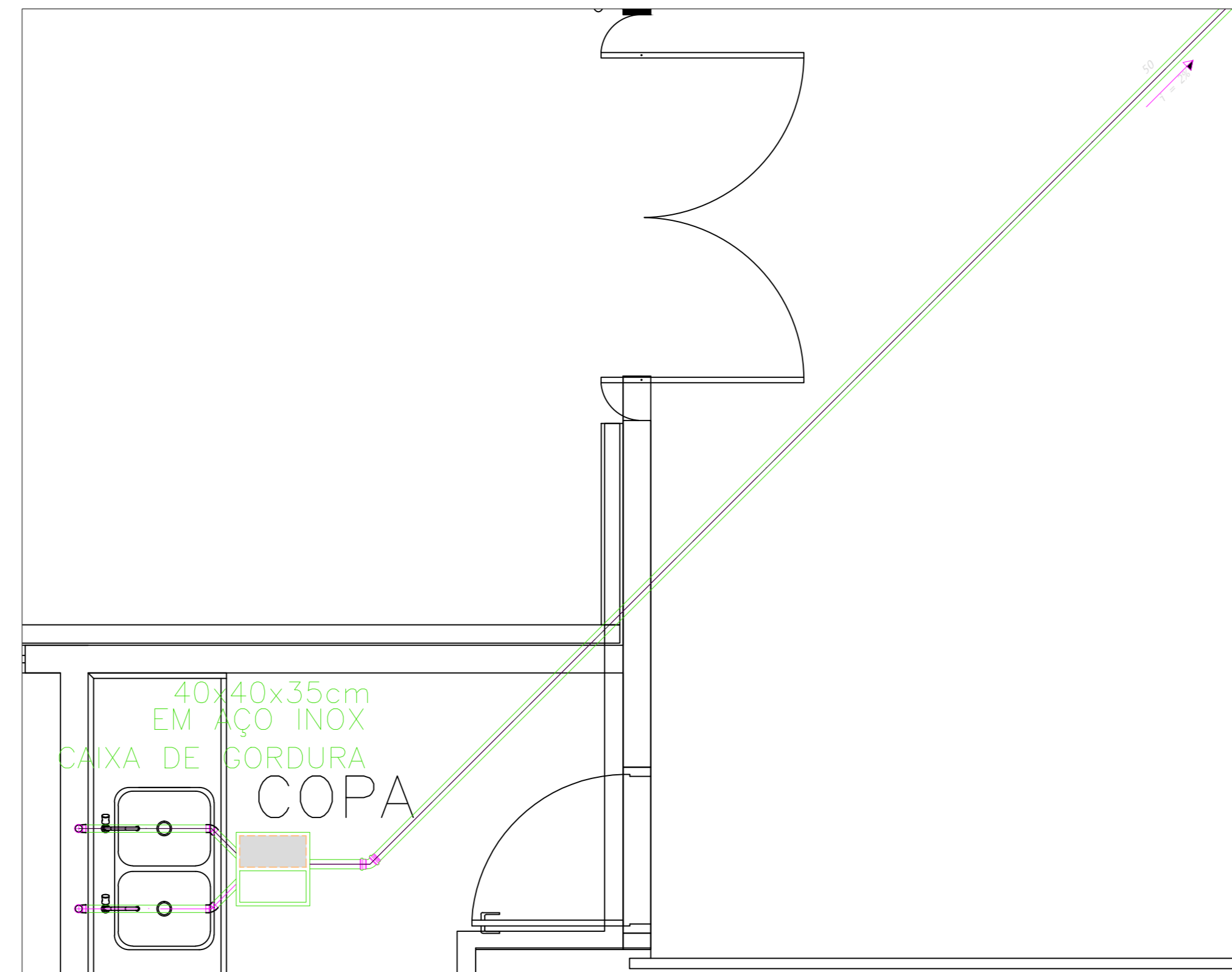
REDE DE ESGOTO DETALHE 1 ESC. 1:25
