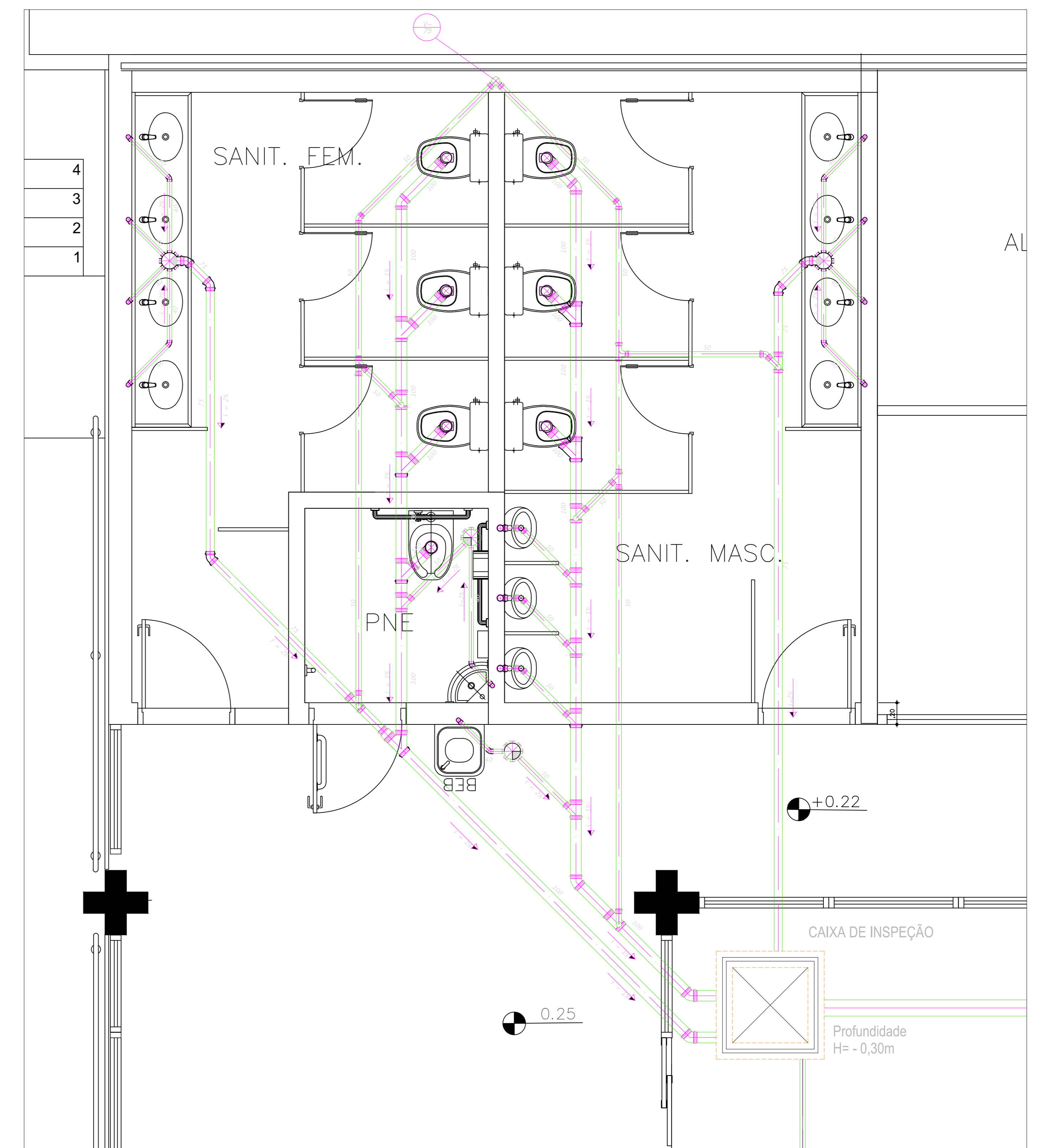
REDE DE ESGOTO DETALHE 1 ESC. 1:25
