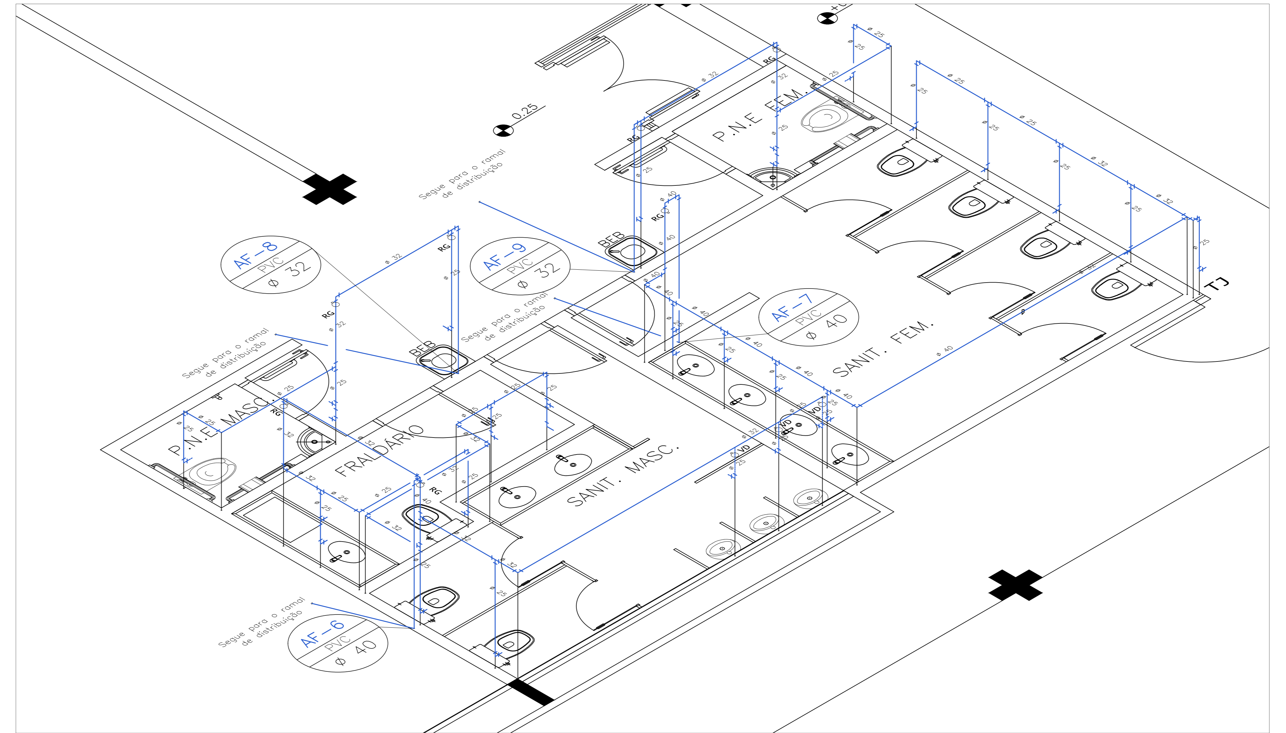
ÁGUA FRIA DETALHE 7 ESC. 1:25
