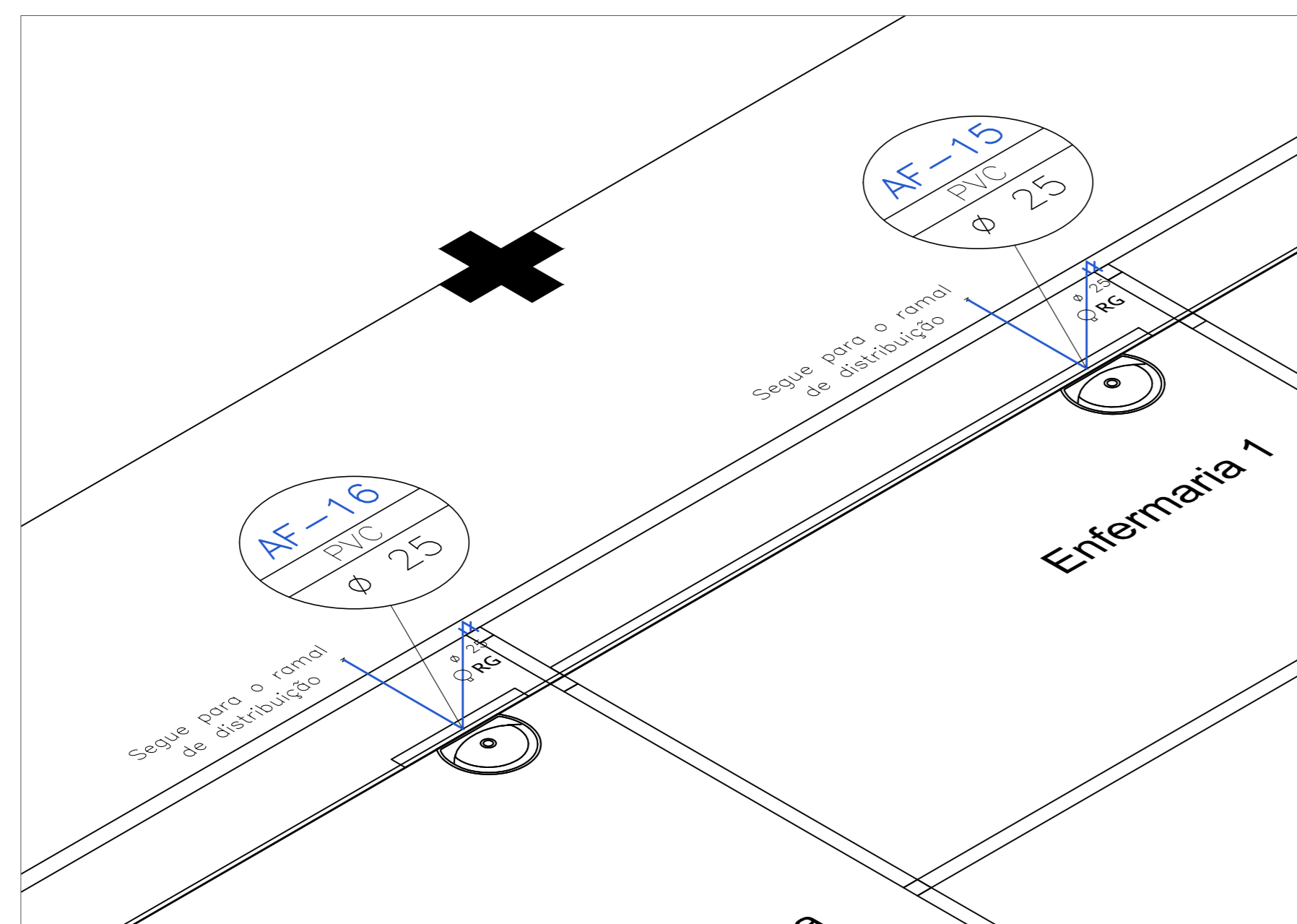
ÁGUA FRIA DETALHE 5 ESC. 1:25
