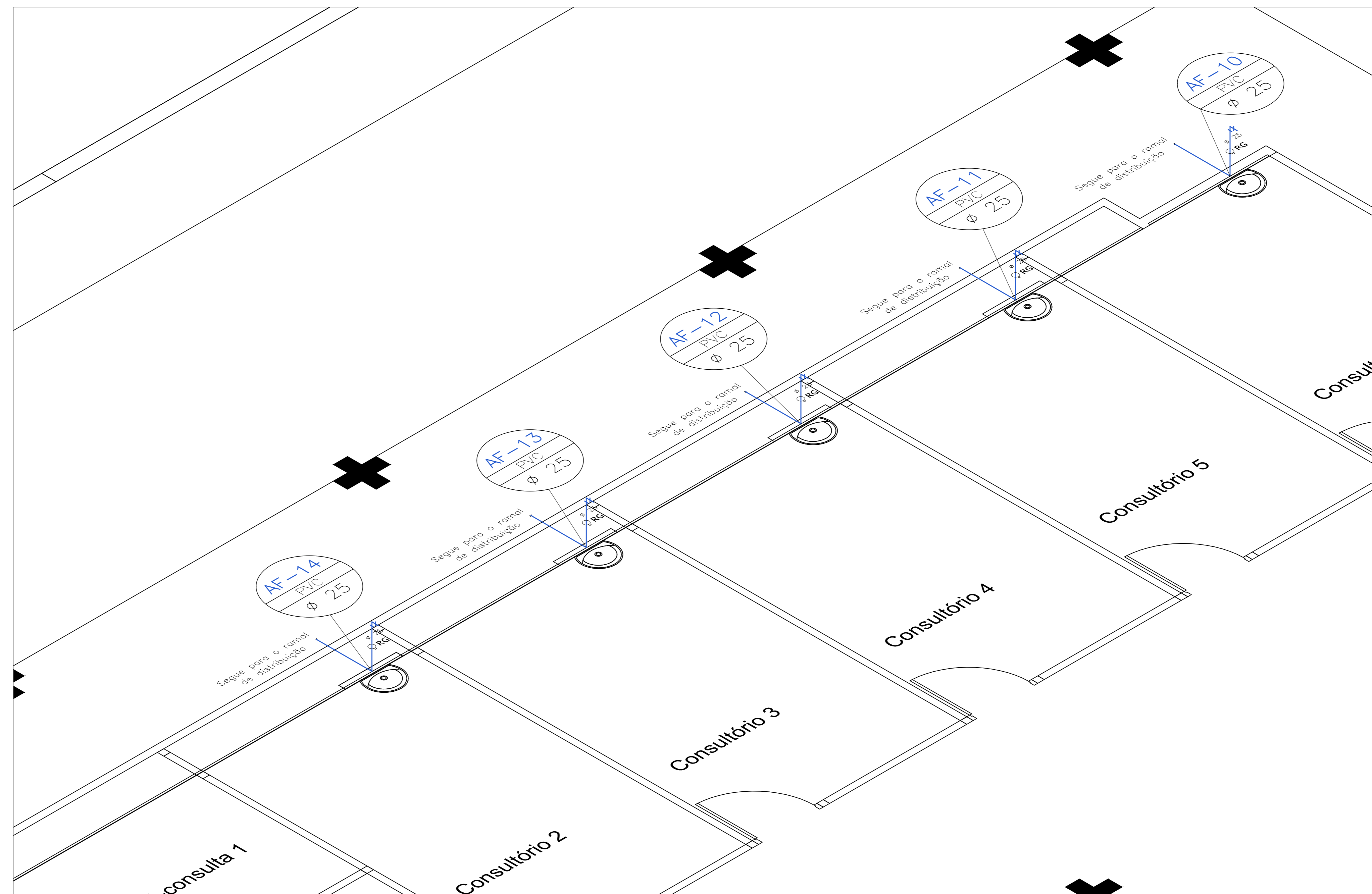
ÁGUA FRIA DETALHE 6 ESC. 1:25
