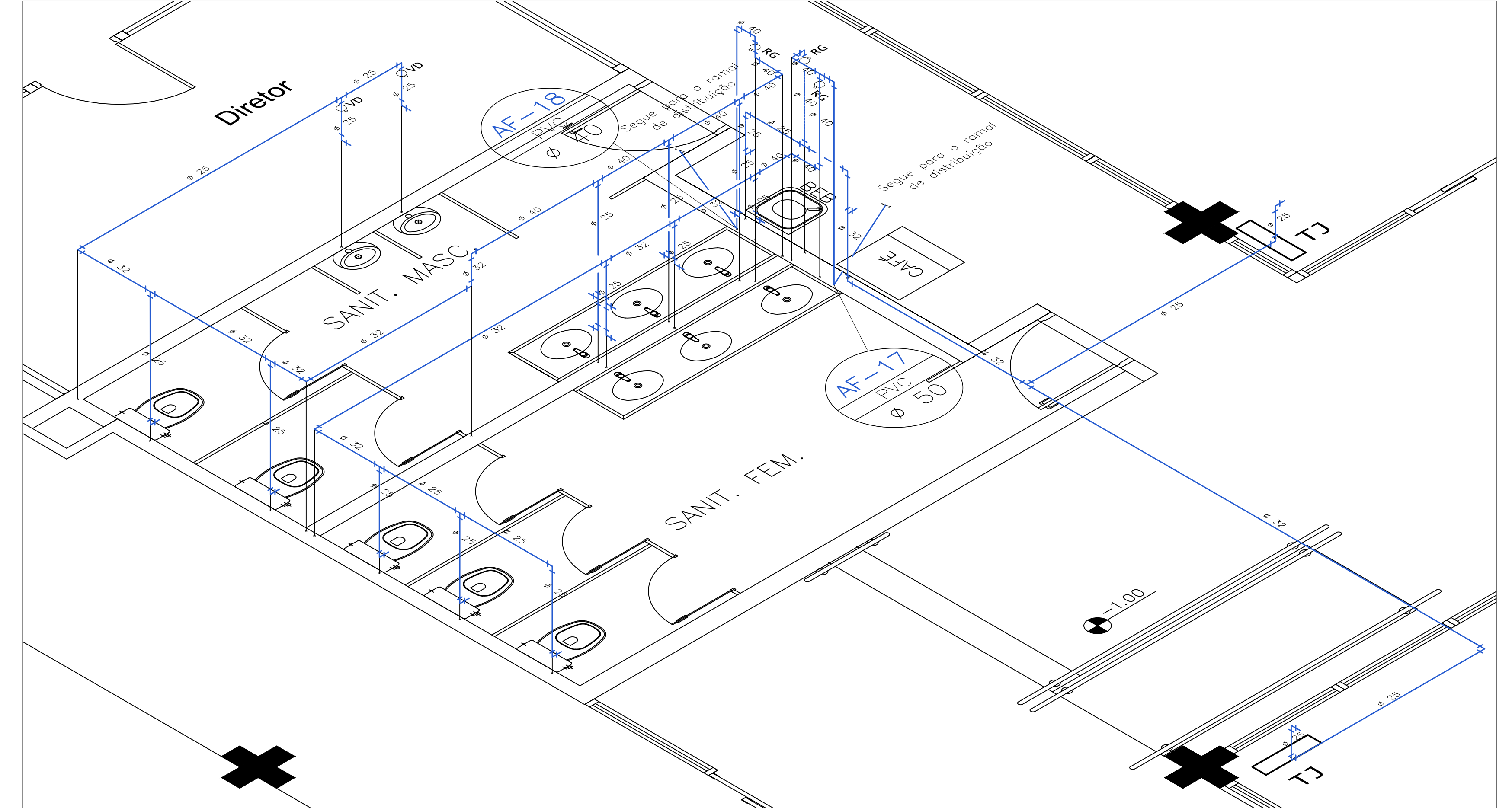
ÁGUA FRIA DETALHE 2 ESC. 1:25
