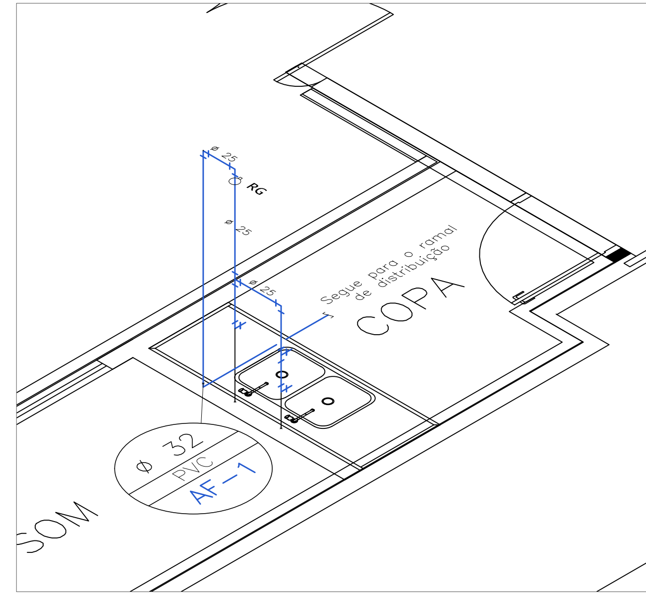
ÁGUA FRIA DETALHE 3 ESC. 1:25
