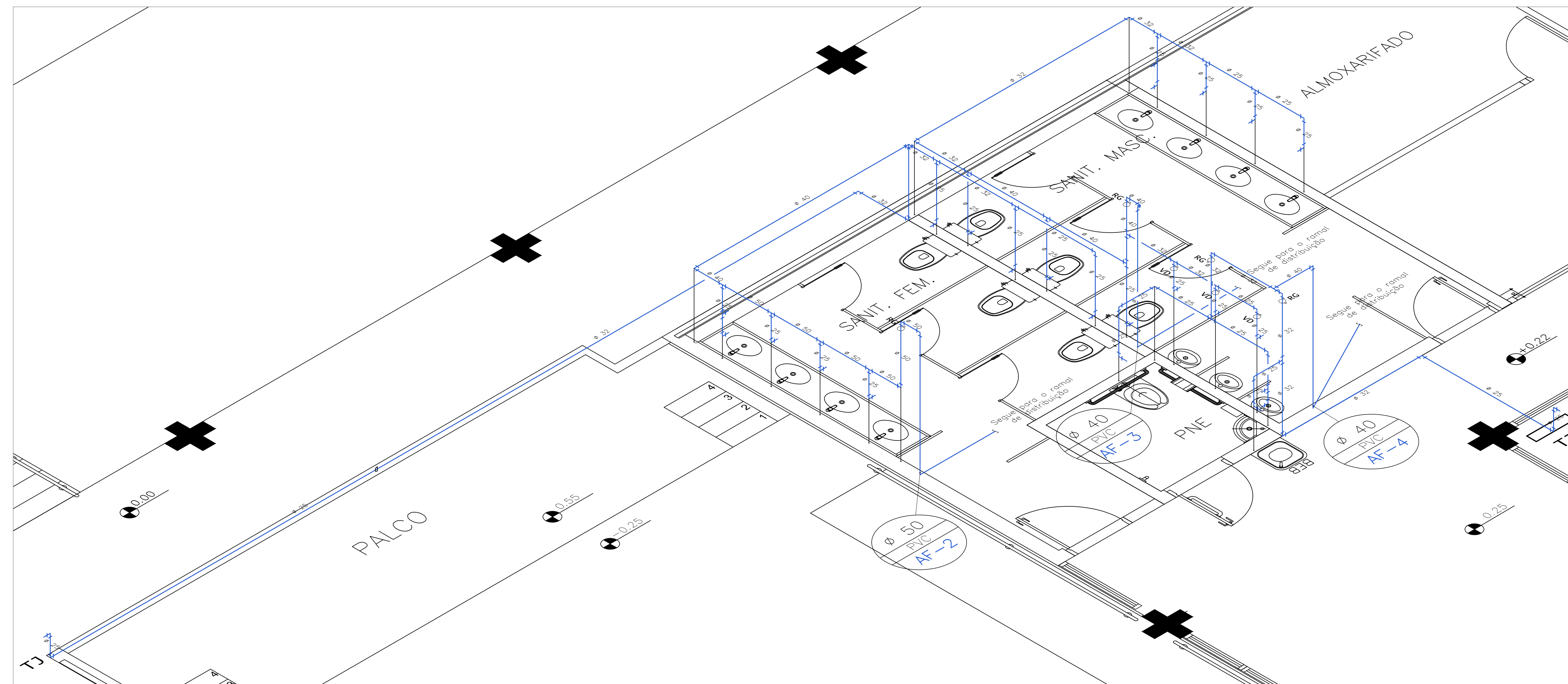
ÁGUA FRIA DETALHE 1 ESC. 1:25
