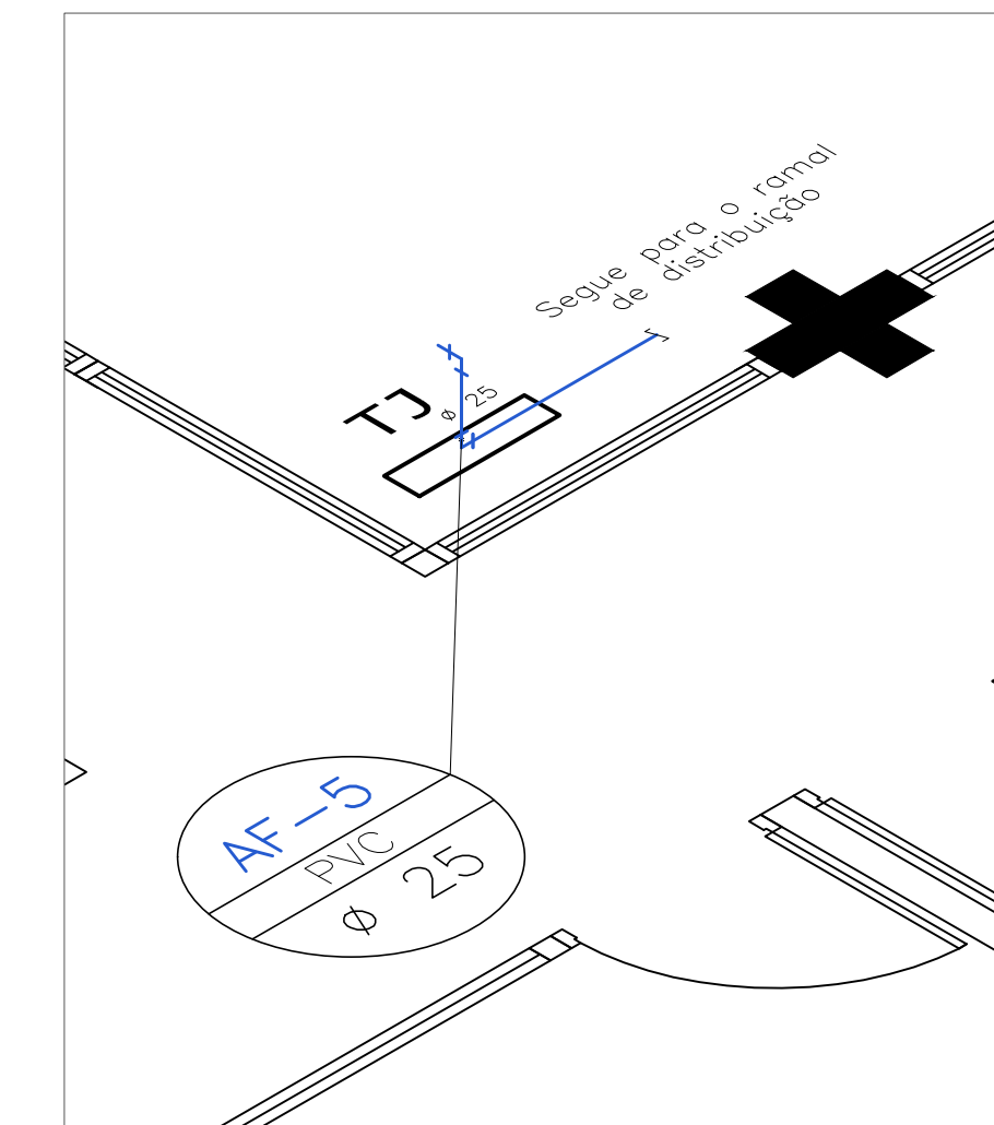
ÁGUA FRIA DETALHE 4 ESC. 1:25
