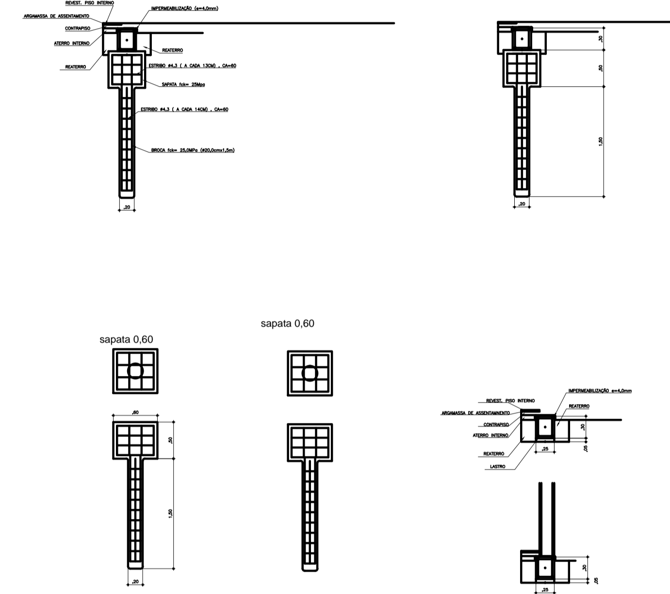
FERRAGENS DET. SAPATA E BALDRAME ESC. 1:50
