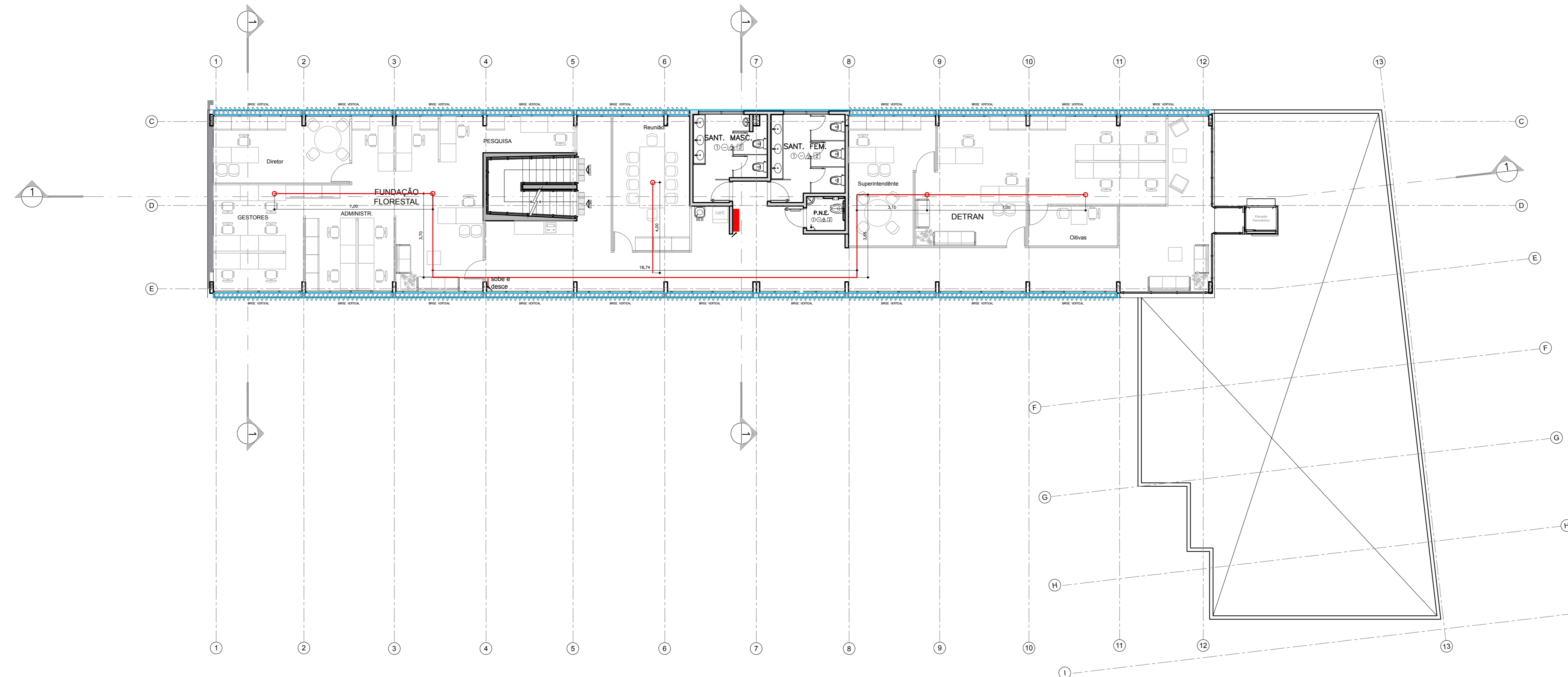
DETECTOR DE FUMAÇA 2. PAVIMENTO ESC. 1:100 ESCALA GRÁFICA
