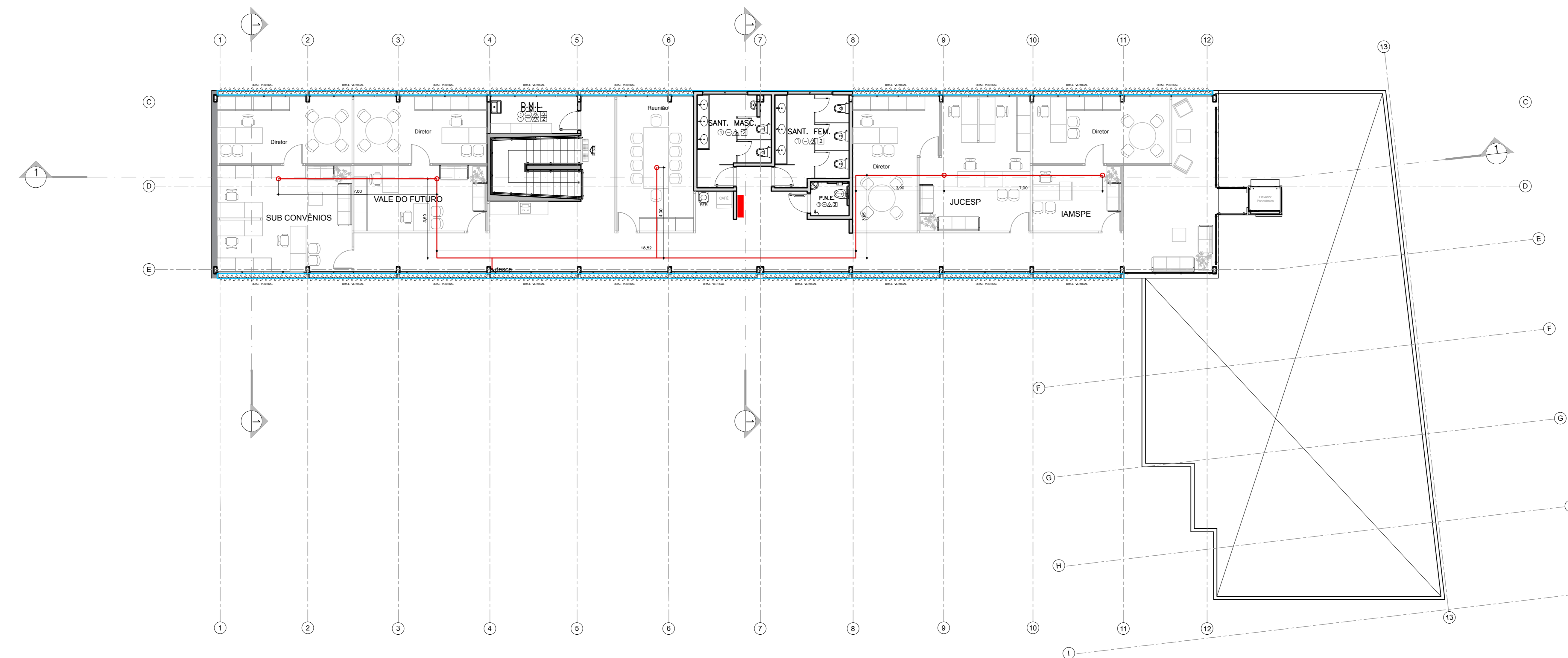
DETECTOR DE FUMAÇA 3. PAVIMENTO ESC. 1:100 ESCALA GRÁFICA
