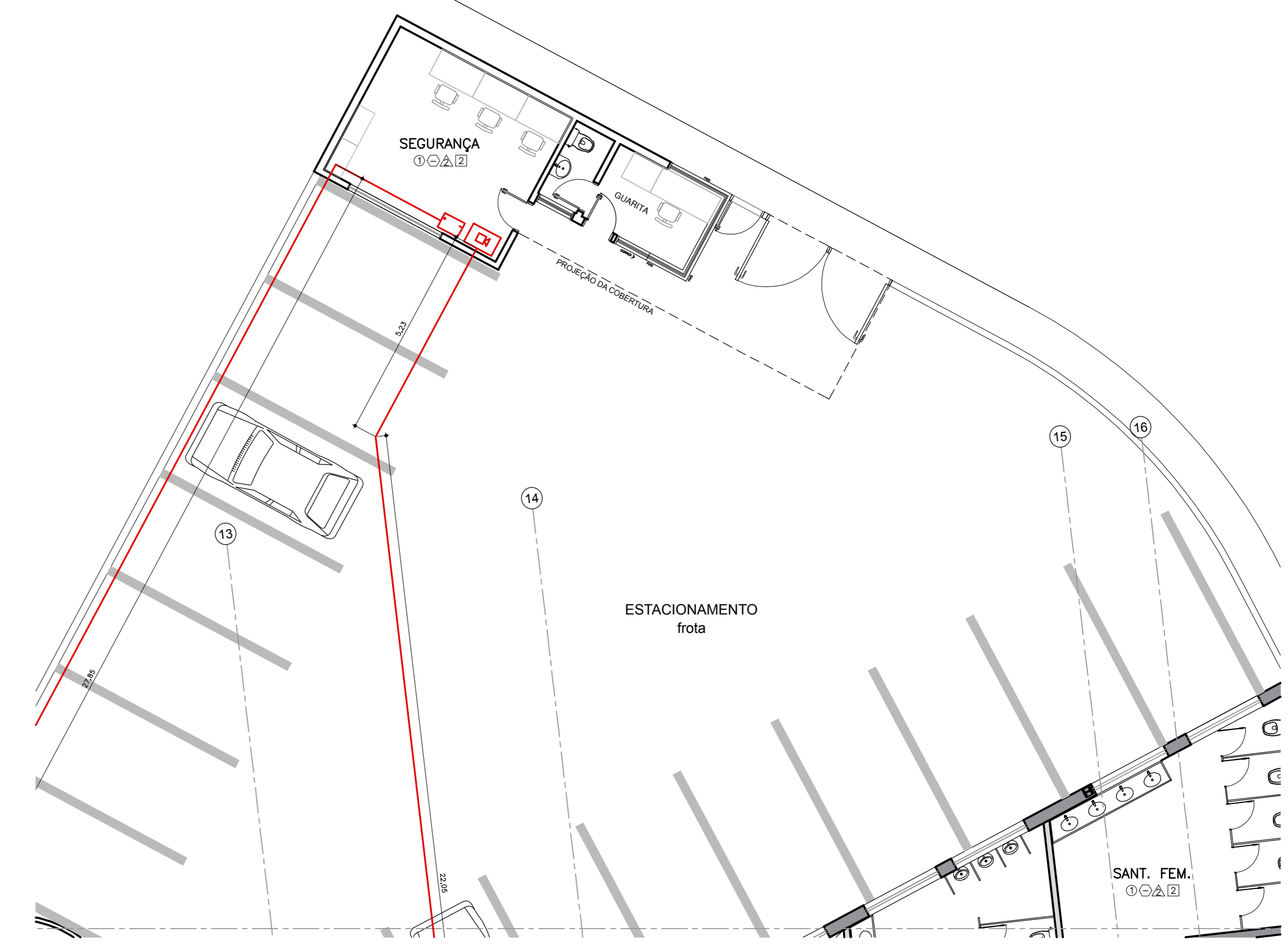
DETECTOR DE FUMAÇA TÉRREO - GUARITA ESC. 1:100 ESCALA GRÁFICA
