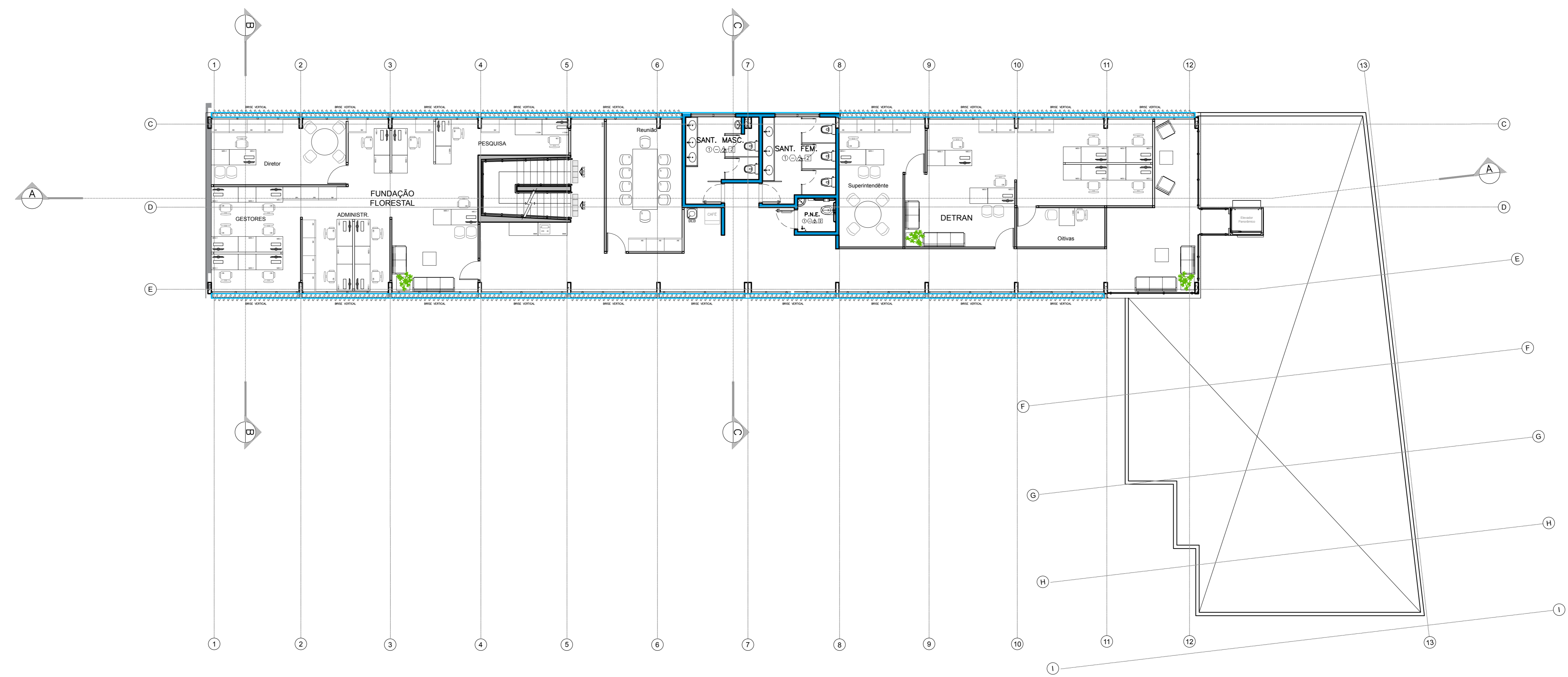
PLANTA BAIXA 2. PAV. ESC. 1:100 ESCALA GRÁFICA
