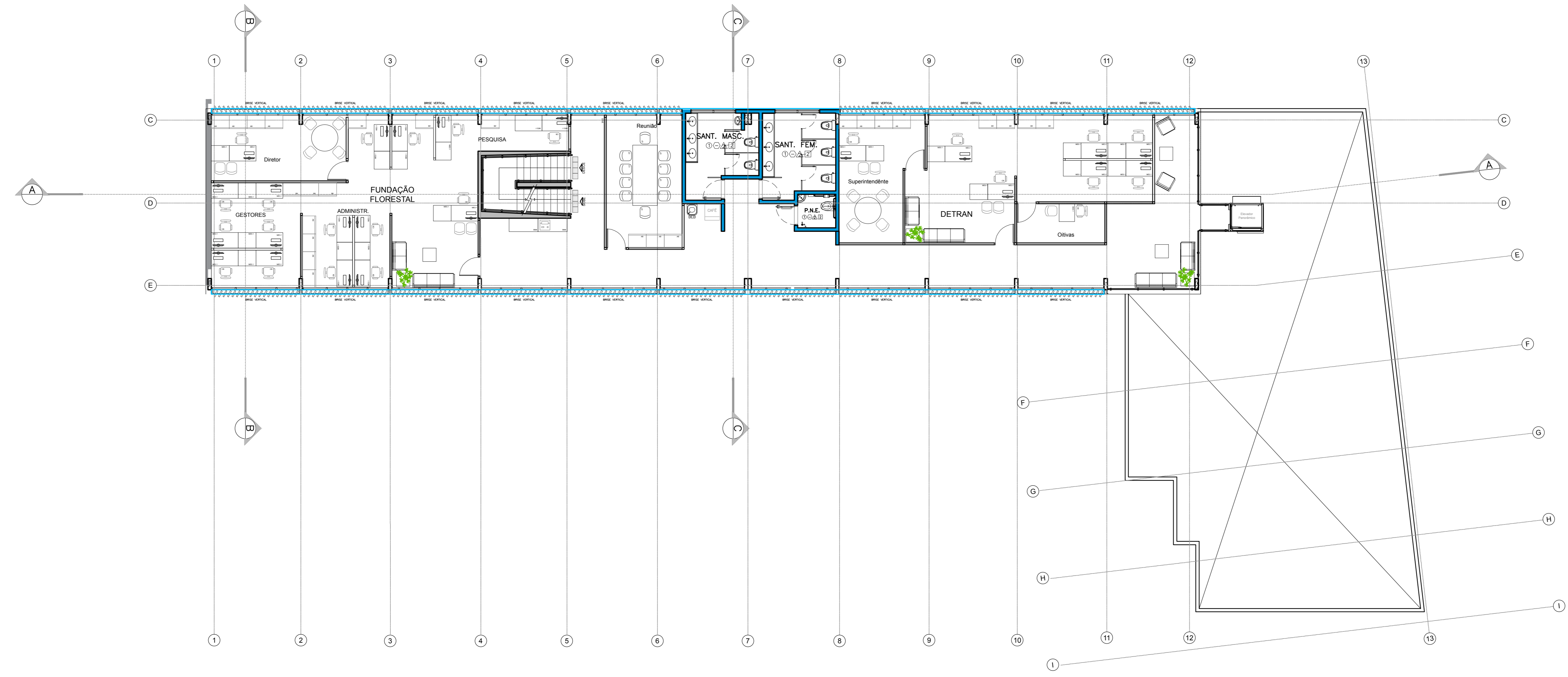
LAYOUT 3. PAV. ESC. 1:100 ESCALA GRÁFICA
