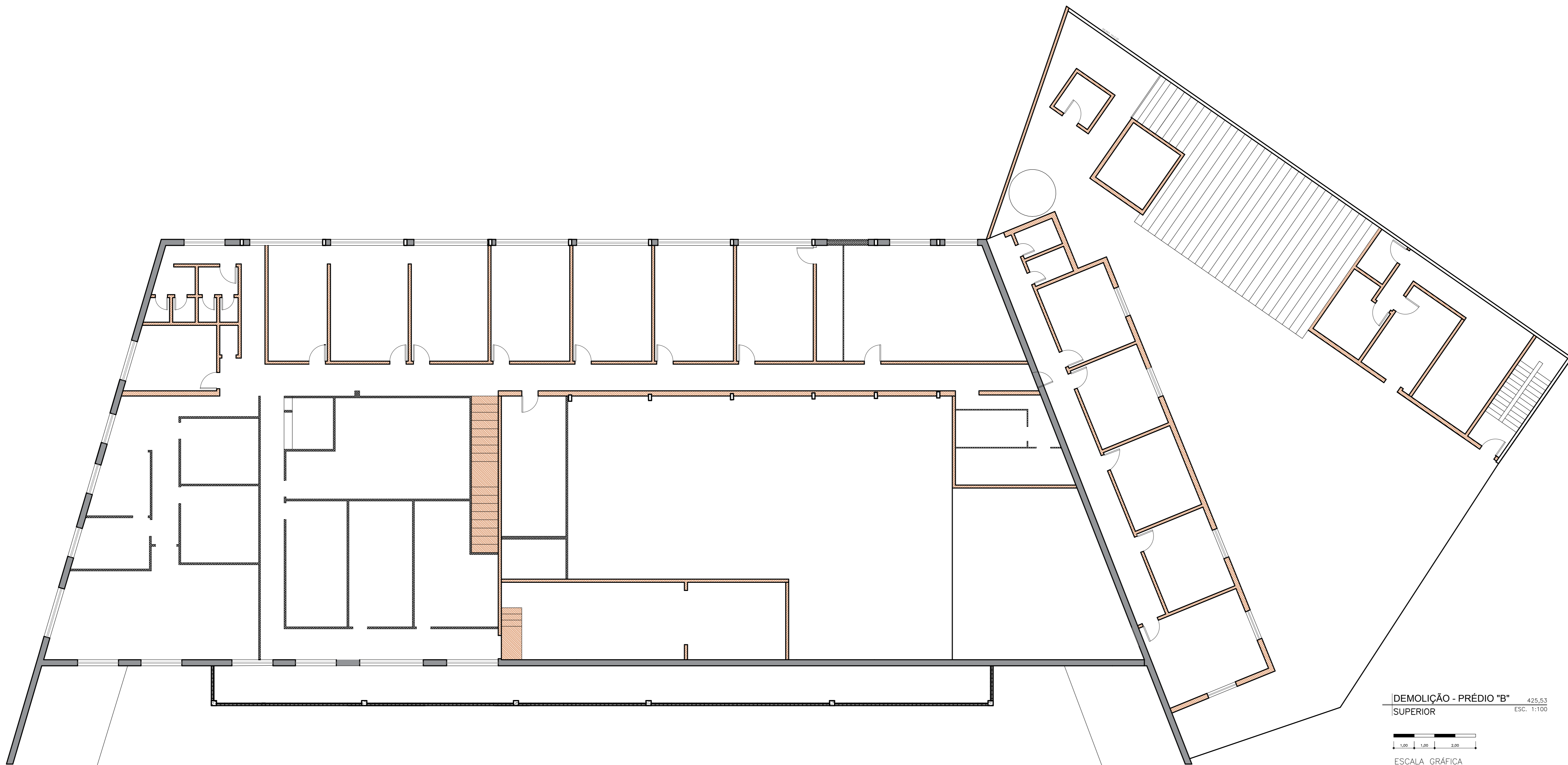
DEMOLIÇÃO - PRÉDIO "B" TÉRRECO 425,53 ESC. 1:100 ESCALA GRÁFICA
