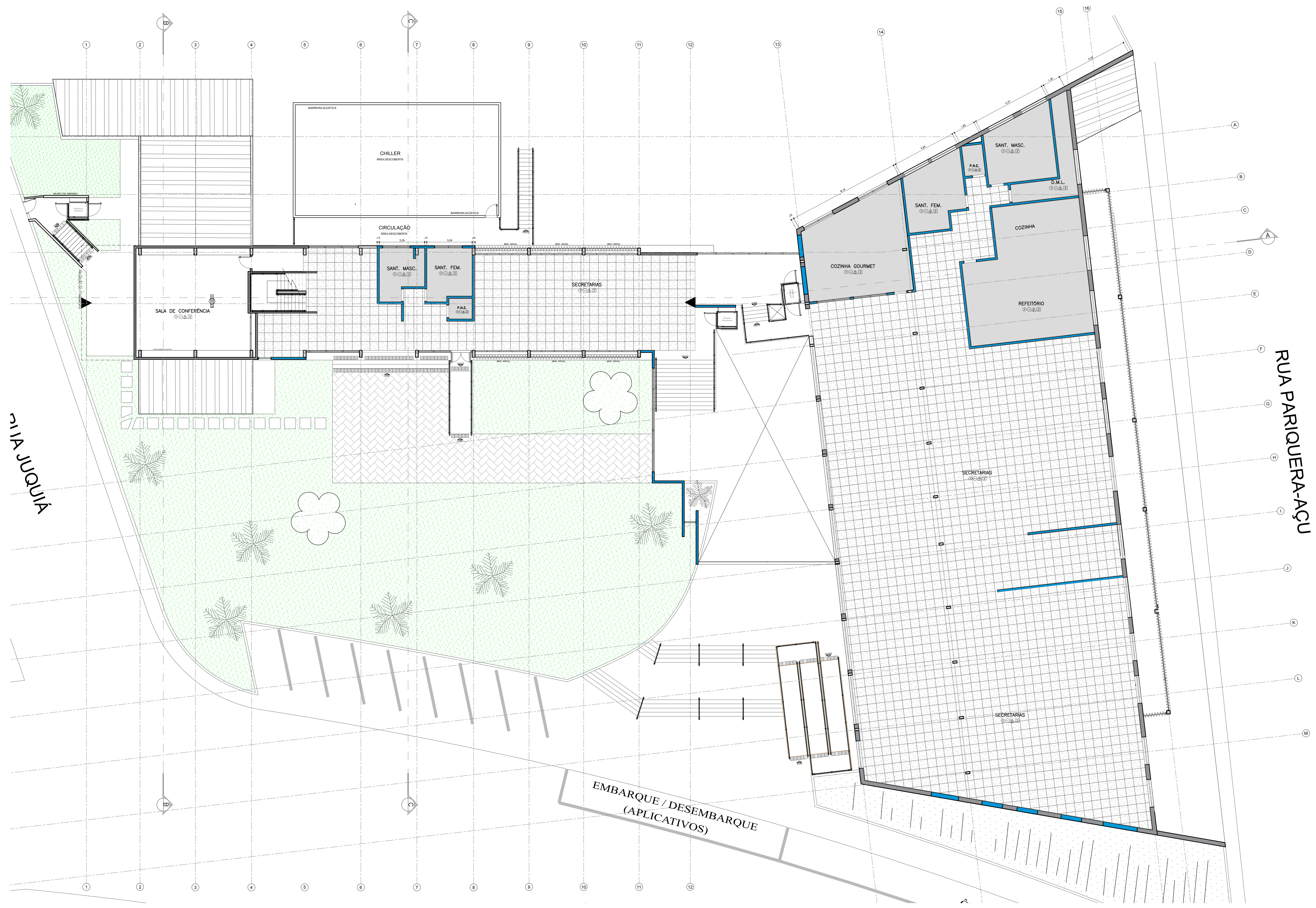
PLANTA DE FORRO 1o. PAV. ESC. 1:100 ESCALA GRÁFICA
