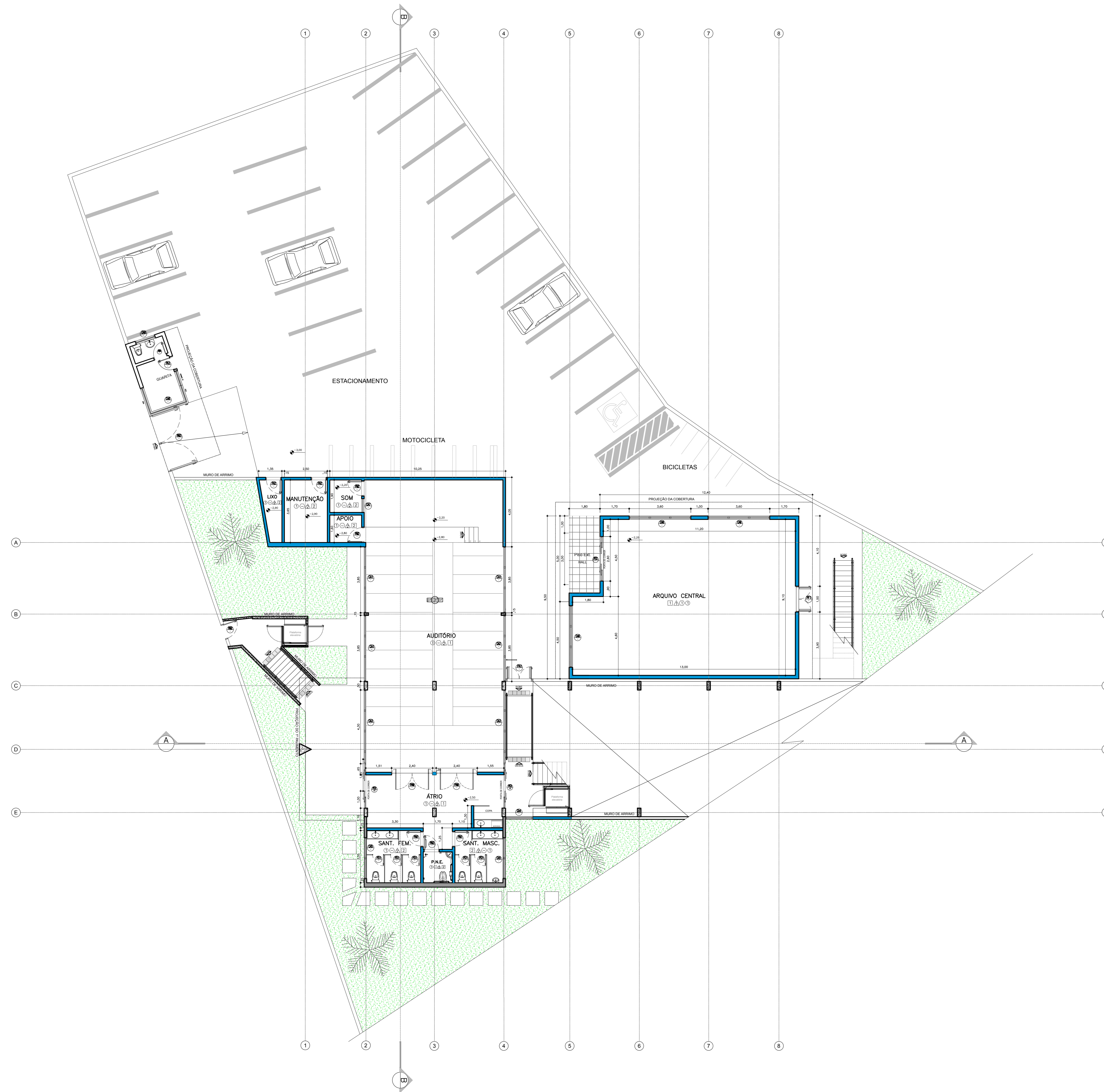
PLANTA BAIXA SUBSOLO 425.53 ESC. 1:1100 ESCALA GRÁFICA
