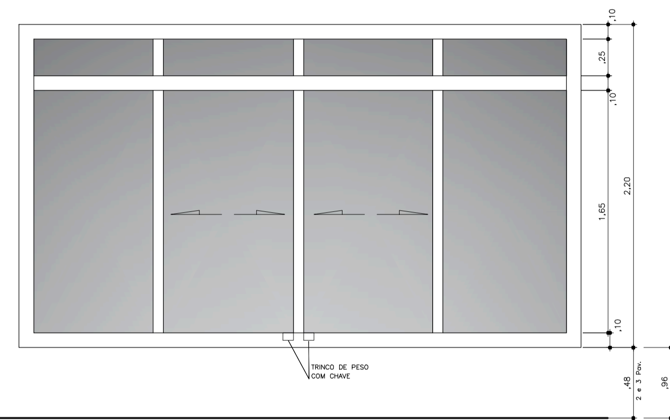
CA22 3,80 x 2,20 ELEVAÇÃO ESC. 1:25
