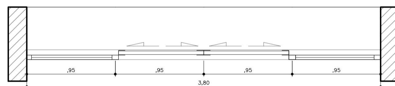
CA17 3,80 x 2,20 PLANTA ESC. 1:25
