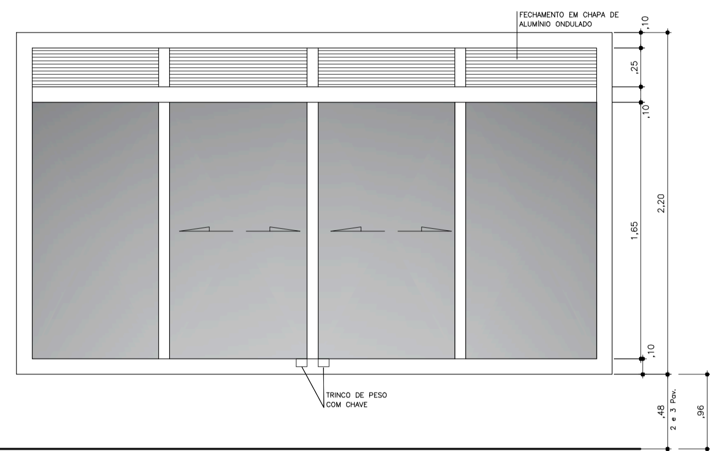
CA17 3,80 x 2,20 ELEVAÇÃO ESC. 1:25
