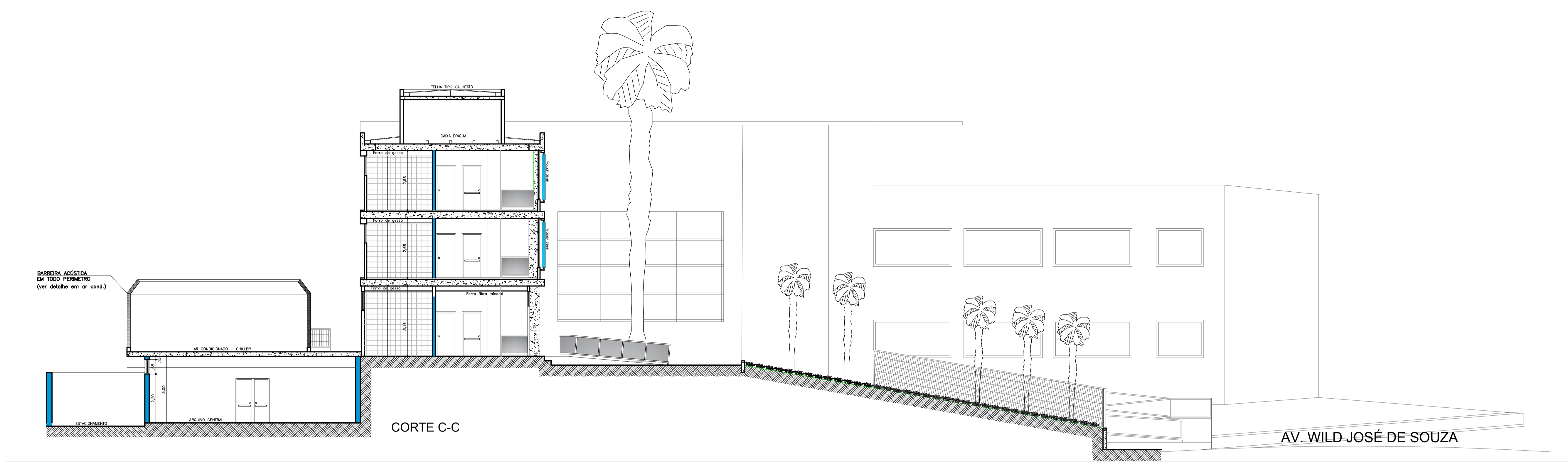
CORTE CORTE B-B ESC. 1:100
