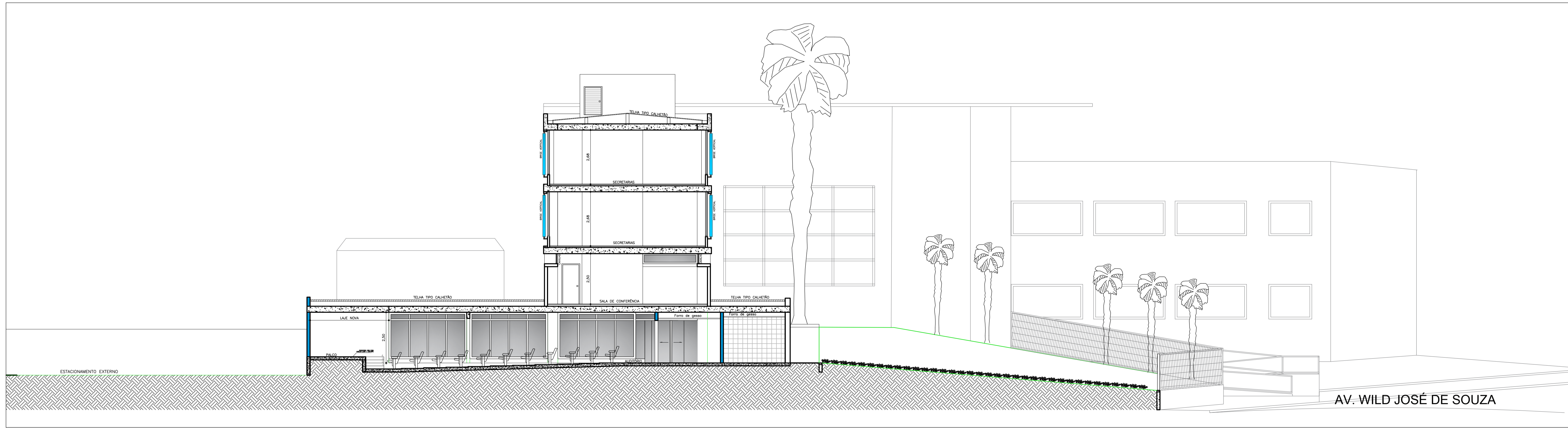
CORTE CORTE C-C ESC. 1:100
